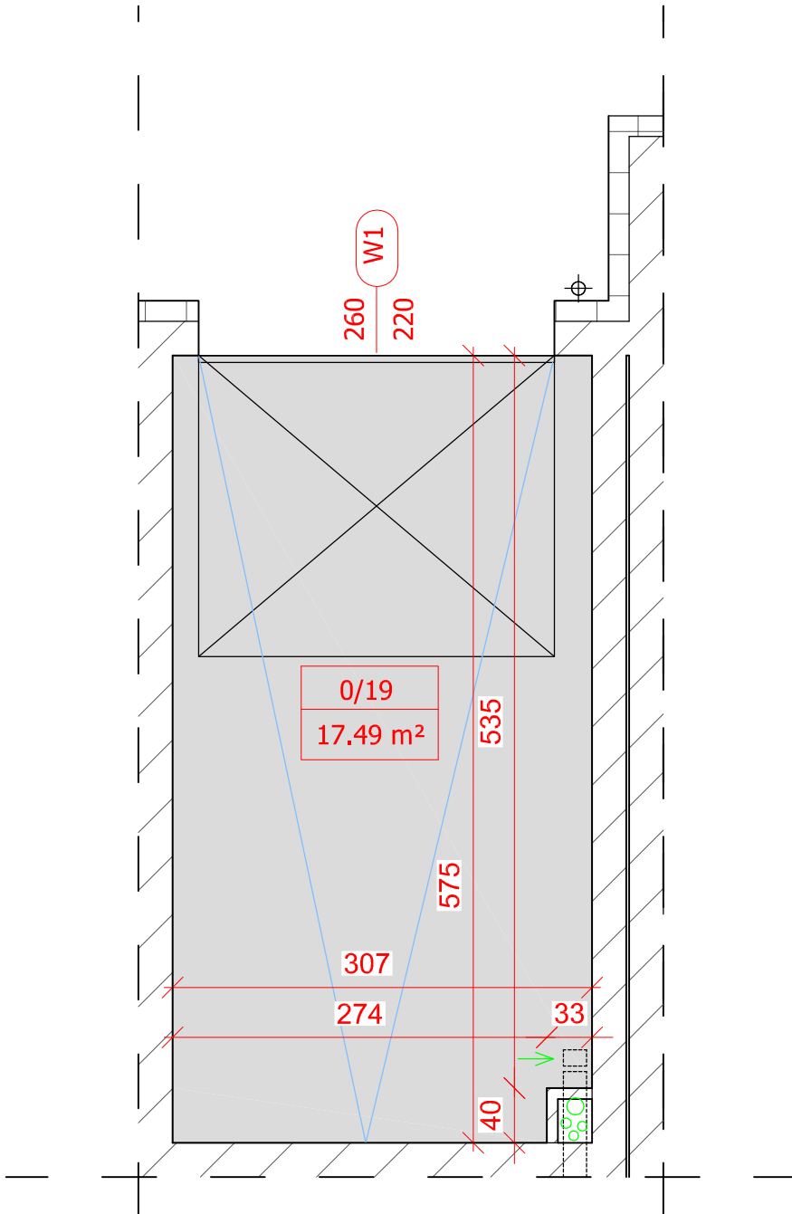
Rzut garażu skala 1:50
